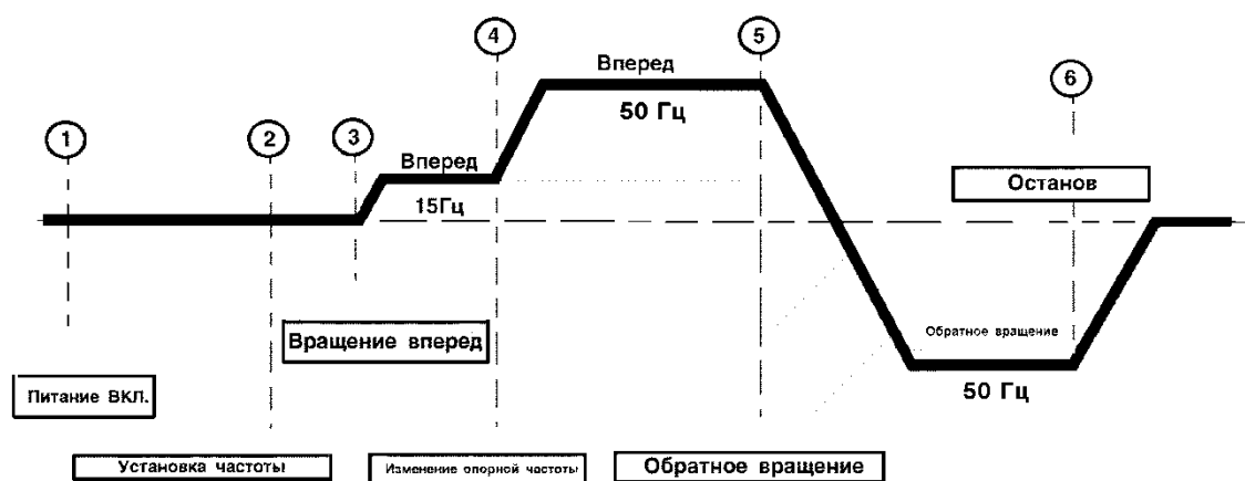
Рис. 15. Последовательность операций при работе с пульта управления.
