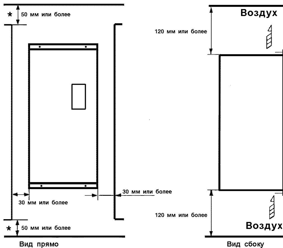
Рис. 8 Расстояния до окружающих устройств.
